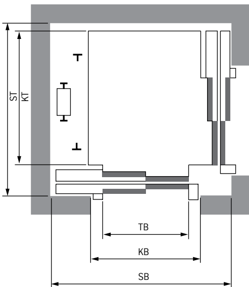
Schachtabmessungen für Übereck- und dreiseitigen Zugang auf Anfrage.
