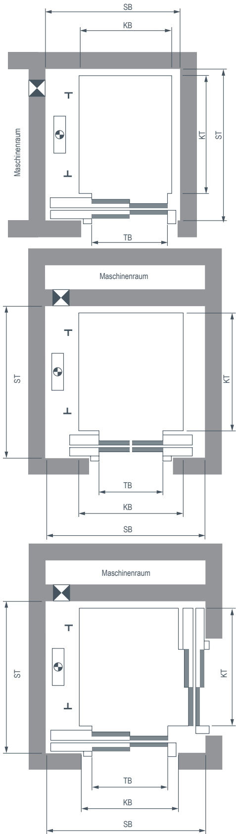
Schachtabmessungen für Übereck- und dreiseitigen Zugang auf Anfrage.
