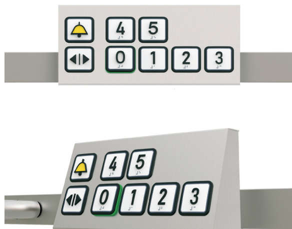
Horizontales Bedientableau 350 × 164 × 92/39 mm
