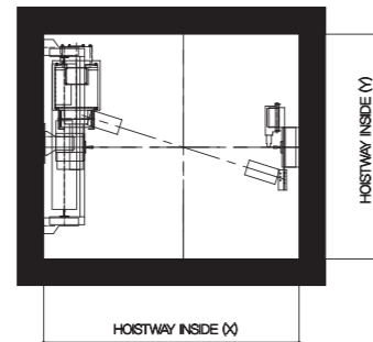
오버헤드 평면도
