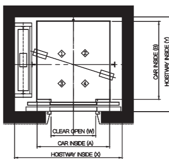
승강로 평면도
