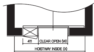
최상층 삼방틀 상세도
