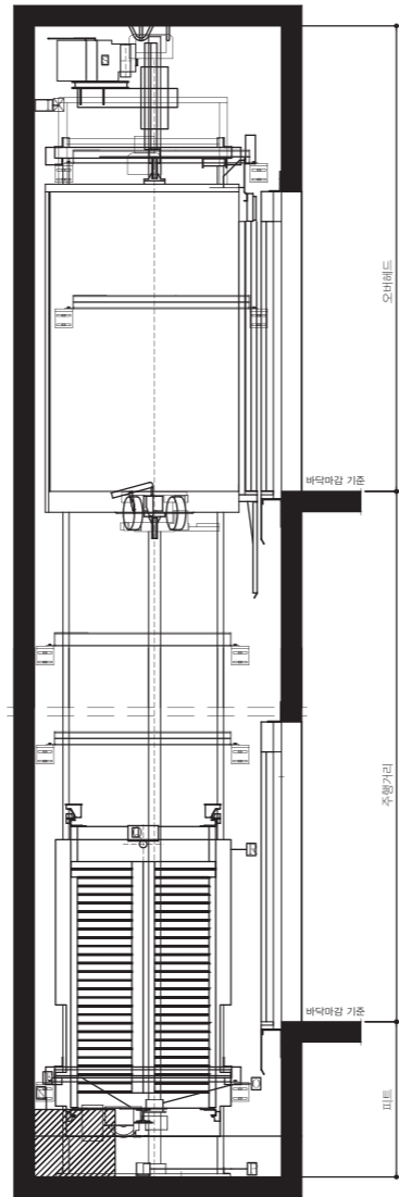
승강로 단면도
