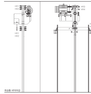
오버헤드 단면도
