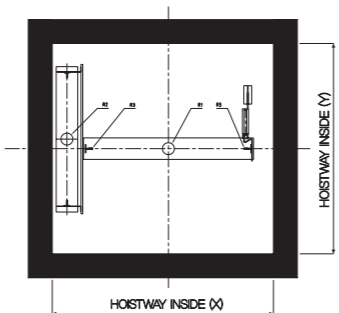
피트 평면도
