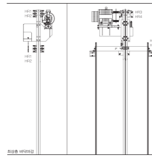
오버헤드 단면도
